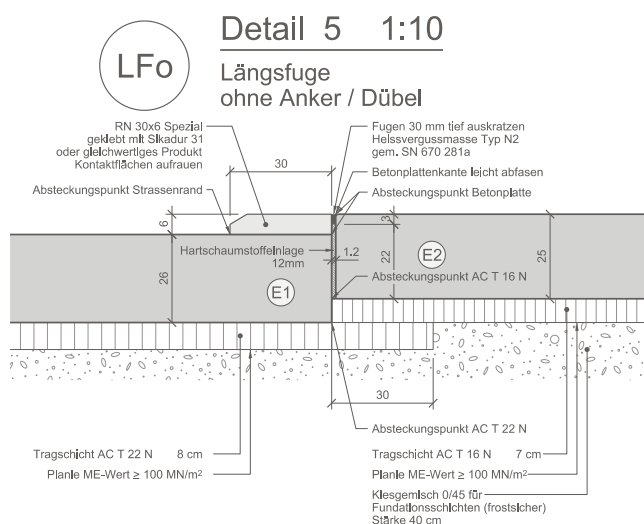
Randabschlüsse Querschnitt, der den Aufbau zeigt.
