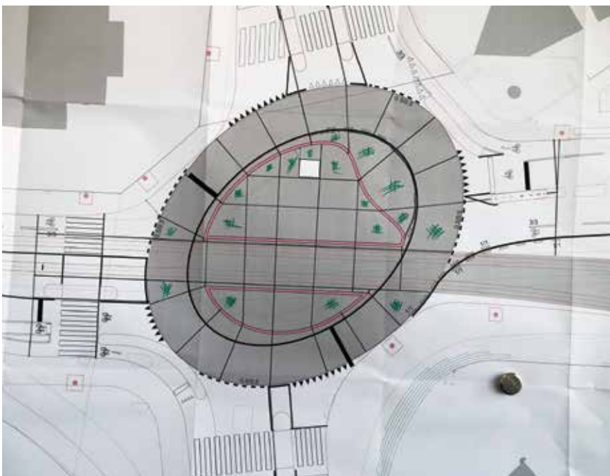
Erste Entwürfe der Fugeneinteilung des Betonkreisells
